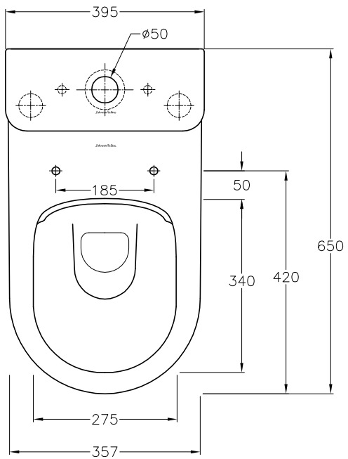
TOP ELEVATION
